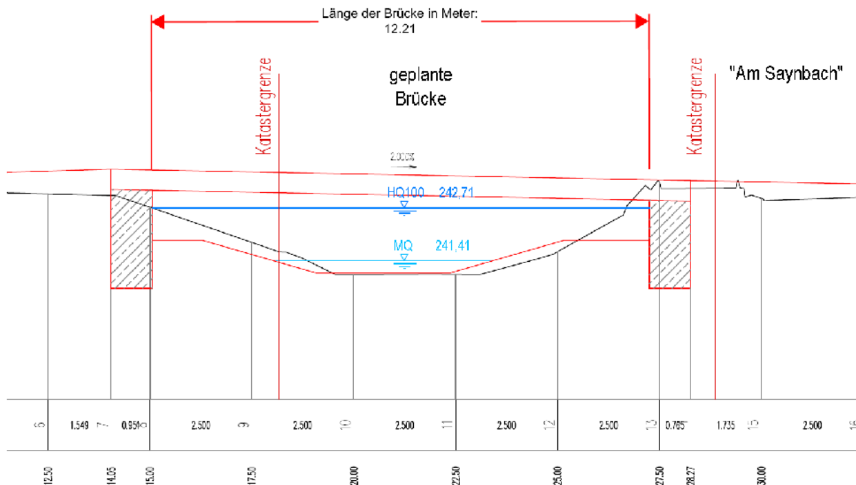
Abbildung 7: Systemschnitt der geplanten Brücke
